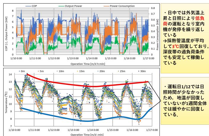
図4 採熱管表面温度とCOPの変化
