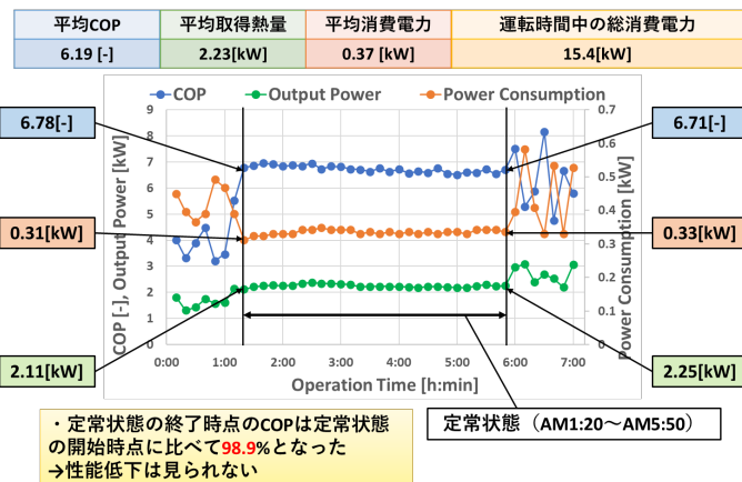
図3 採熱管表面温度と水温との温度差, COPの変化
